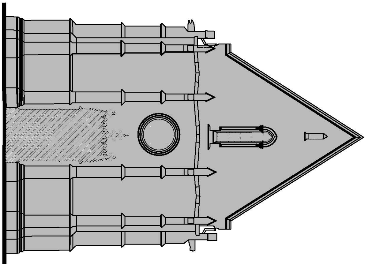
FACADE OUEST - WESTGEVEL
